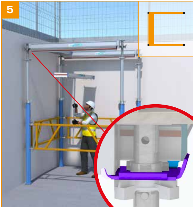
- Mise en place des panneaux Eco+ à l'aide de la TopPerche. Attention : les dents extérieures du panneau Eco+ doivent impérativement reposer sur une poutrelle primaire ou sur la tête d'étais.
