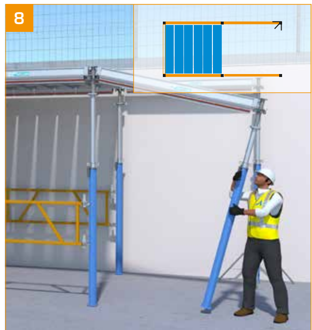
- Le poseur se sert de l'étau pour placer la poutrelle primaire.
