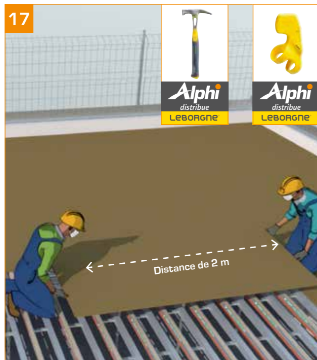
- Quand la structure est terminée et réglée en hauteur : mise en place du contre-plaqué (CP). - Utilisation de la servante pour le découpage du contre-plaqué (voir Accessoires p. 9-10). → Sécurité périphérique (voile, poutre...) réalisée au préalable. → Utilisation de la servante pour découpe contre-plaqué.
