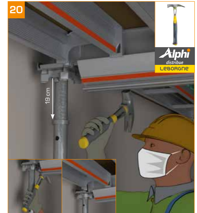
- Décoffrage de la dalle : décinturer les têtes coffrantes des ST à l'avancement. - Les poutrelles primaires et les cadres C2+ ou C4+ descendent de 19 cm. - Les ST restent en place.
