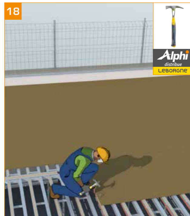
- Clouage avec des pointes de 40 mm maximum. - S'assurer de la présence d'un porteur sous le joint des feuilles de CP. - S'assurer de l'étanchéité du coffrage entre feuilles de CP et à la périphérie. Interdiction de circuler sur les panneaux de contre-plaqué, sauf pour le personnel formé et habilité à poser les panneaux de contre-plaqué.
