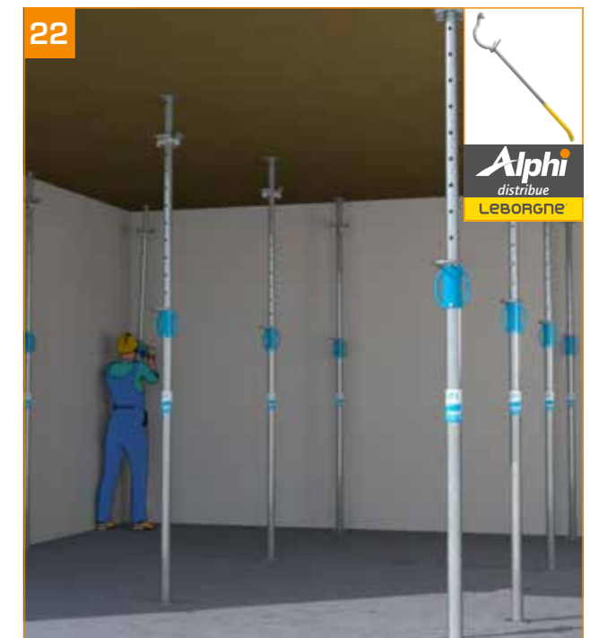
- Décoffrage de la dalle : enlever les ST placés en périphérie des cellules. - Laisser en place pendant 3 jours minimum les autres ST (selon type de béton et température extérieure).
