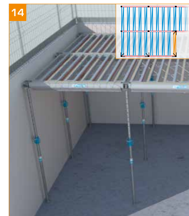
14 - Continuer l'avancement des cadres C2+ à l'aide de la TopPerche, ou C4+ de proche en proche.
